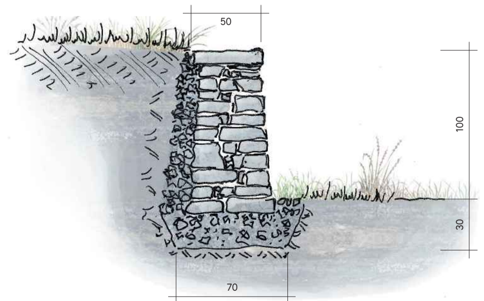
Stützmauer
